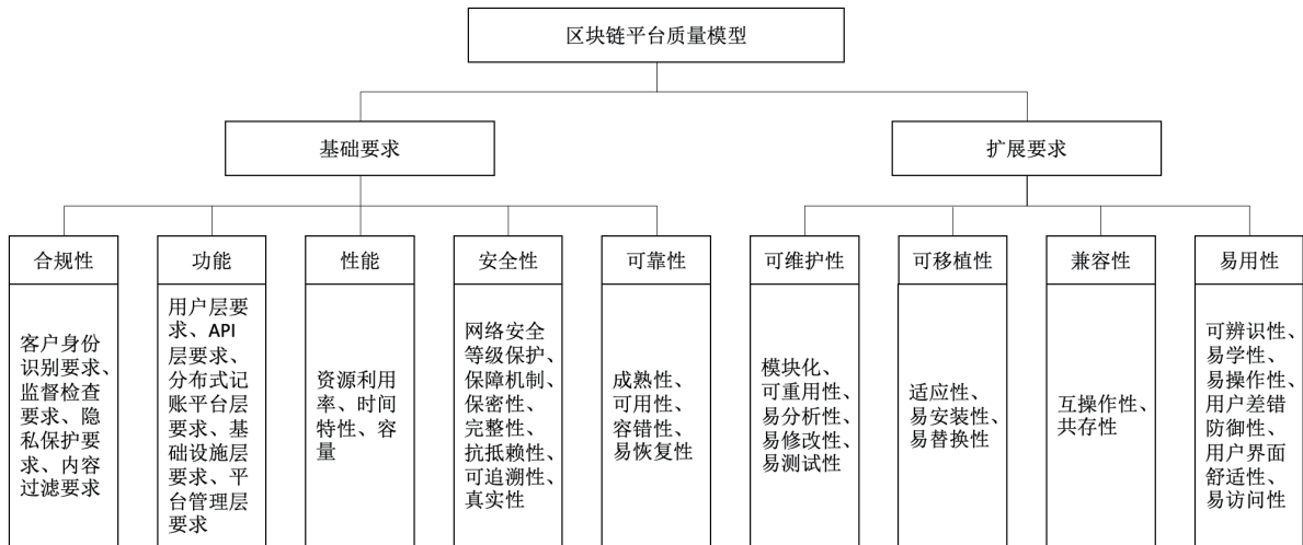
区块链平台质量模型
